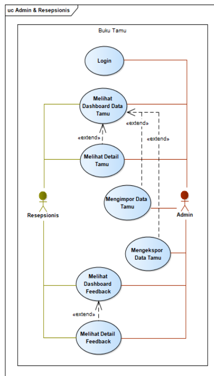
Gambar 3. Usecase Diagram (Admin dan Resepsionis)
